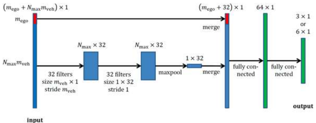
Figur 16. Arkitekturen för det neurala nätverket (Hoel, 2021).
