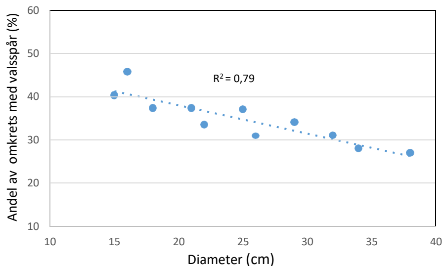
Figur 4. Andel av omkretsen med synliga spår av skördaraggregatets (H415) matarvalsar på 11 stockar från olika träd vid avverkningen Fjällnora I. R^2 =determinationskoefficient
