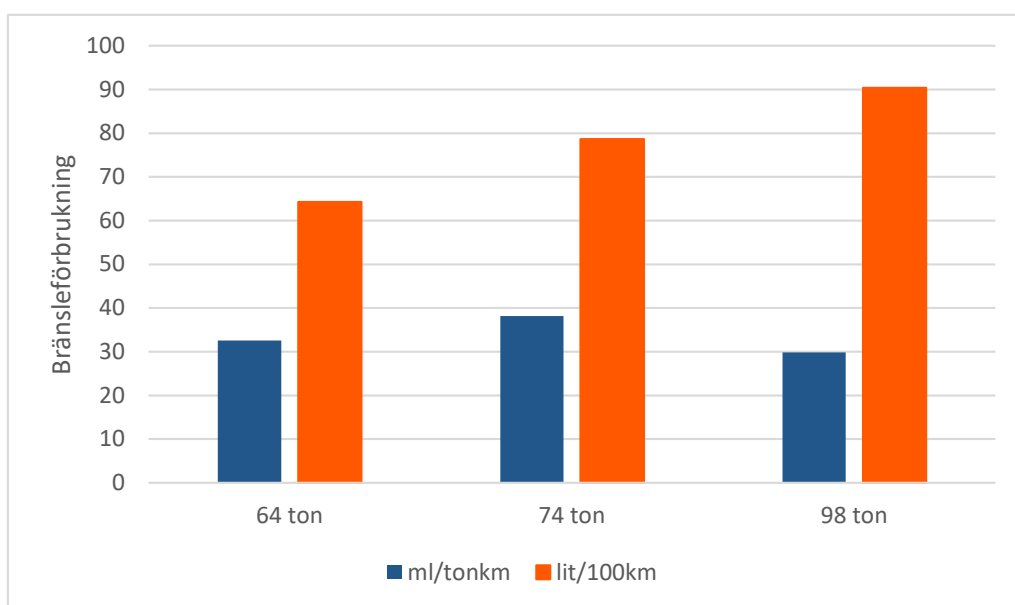
Figur 10. Bränsleförbrukning per tonkm respektive 100 km beroende av fordonsstorlek.
