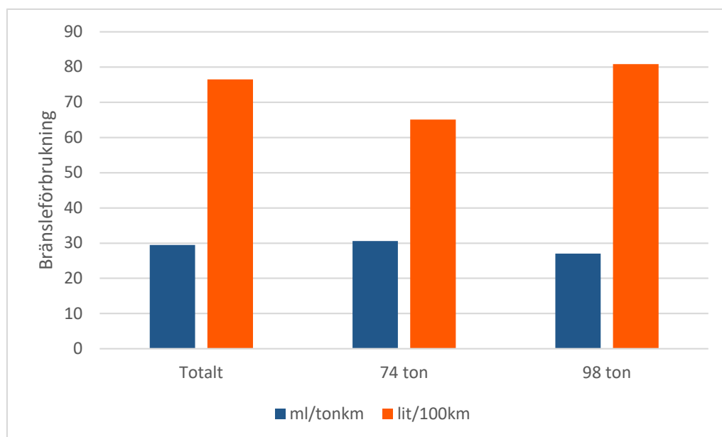
Figur 7. Bränsleförbrukning per tonkm respektive 100 km beroende av fordonsstorlek. Totalt är fordonskombinationerna tillsammans.
