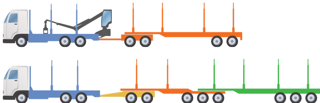
Figur 1. Jämförelse mellan en 60 (64) tons timmerbil på ca 22 meter och det 30 meter långa ETT-fordonet på 90 ton.
