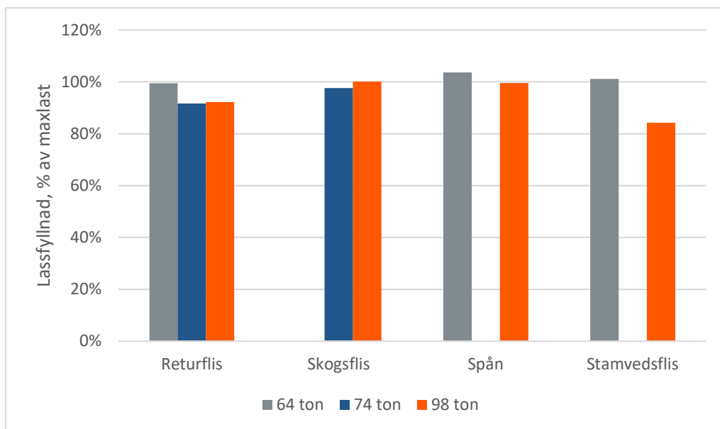
Figur 9. Genomsnittlig lassfyllnadsgrad beroende av fordonskombination och transporterat material. Det mindre 64-tonsfordonet har till stor del kört blöt flis, därav den höga lassfyllnaden.
