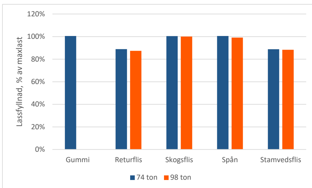
Figur 5. Genomsnittlig lassfyllnadsgrad beroende av fordonskombination och transporterat material.
