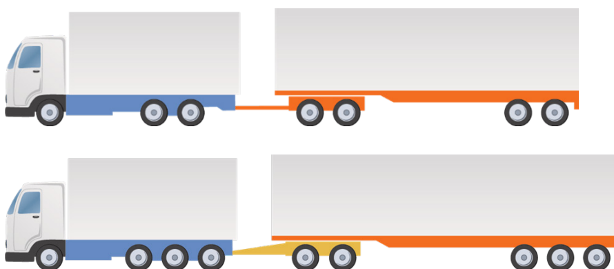
Figur 2. Försöksfordonet i nioaxligt utförande med en tillåten bruttovikt om 74 ton nederst i jämförelse med ett sjuaxligt 60 (64)-tonsfordon överst.
