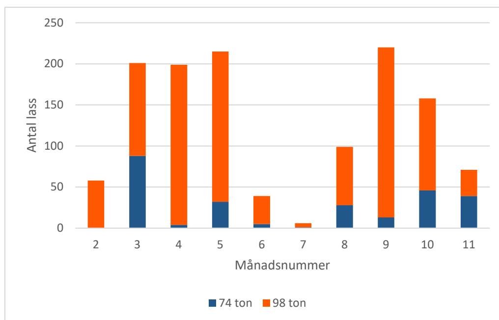
Figur 4. Antal lass per bruttovikt och månad för de två kombinationerna.
