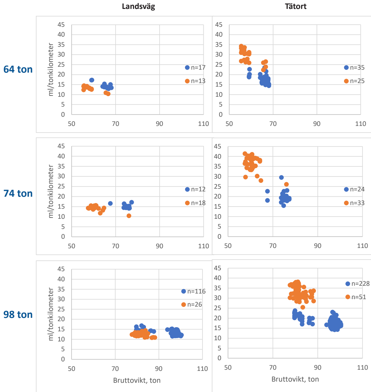
Figur 12. Bränsleförbrukning uttryckt som ml/tonkilometer för de tre fordonskombinationerna. Blått innebär transport mot Igelstaverket med i huvudsak nedförskörning och orange är transport upp mot Nykvarn. Diagrammen i den vänstra kolumnen är landsvägskörning och i den högra kolumnen tätortskörning (n = antalet datapunkter per serie/färg).
