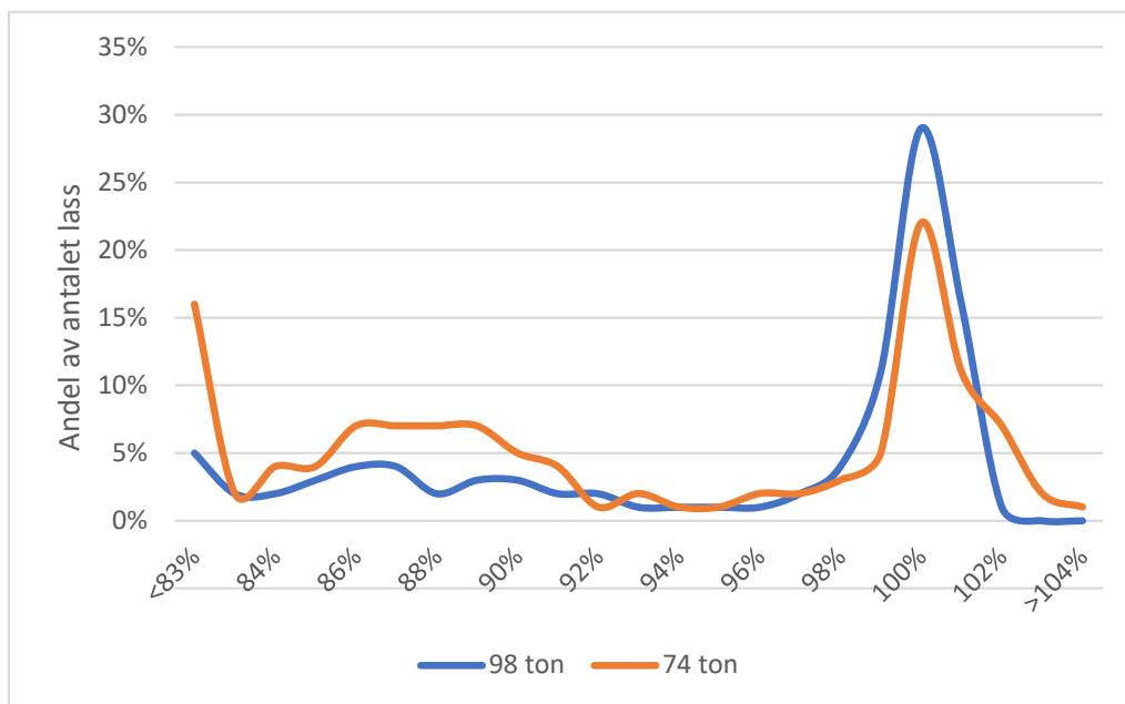
Figur 6. Andel lass per lassfyllnadsgrad för de bägge fordonskombinationerna. Den topp som bildats kring < 83 procent lassfyllnad beror på att en del lass gått med mycket lätta material.
